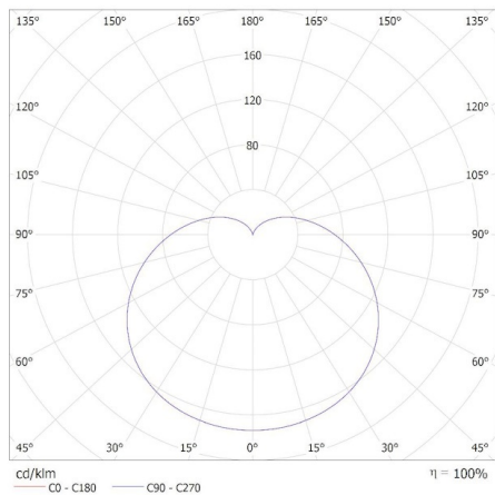
KANLUX S.A. (kat 26767) BILO 6,5W E14-WW / Krzywa rozsytu światła (biegunowo)
