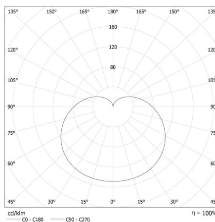
KANLUX S.A. (kat 33718) IQ-LED A60 9,6W-CW / LDC (Polar)
