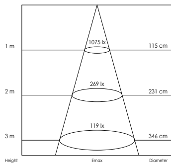
DIAGRAM NA ZÁKLADĚ 411070X0 (3000K) DIAGRAMS BASED ON 411070X0 (3000K)
