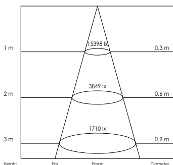
DIAGRAM NA ZÁKLADĚ 41101X30 (3000K, 20°, RA>90) DIAGRAMS BASED ON 41101X30 (3000K, 20°, RA>90)
