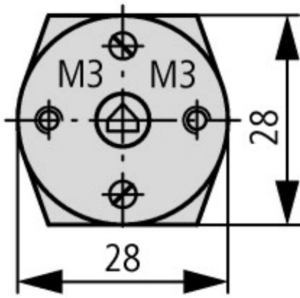
Rozměry otvorů dveří
