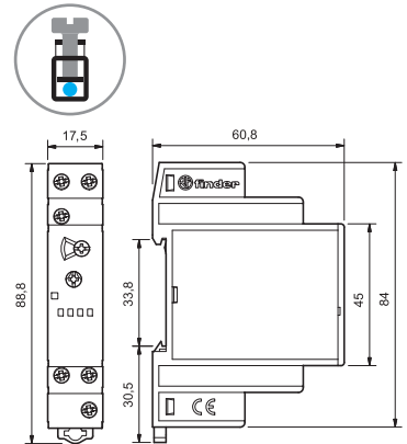
80.71 šroubové svorky
