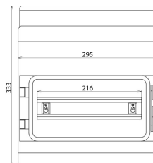
Rozměry IGA 12 IP65
